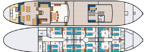
Decks- und Kabinenplan LEAFDE FAN FRYSLAN
